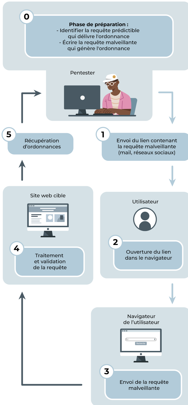
Exemple de vulnérabilité (CSRF) pour la délivrance d'ordonnances
